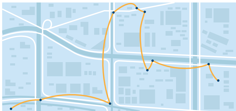
图4.2.12 行动轨迹
