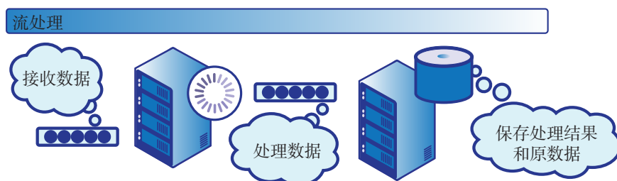
图4.1.13 流处理
