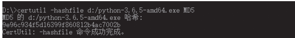
图3.1.5 计算MD5值
