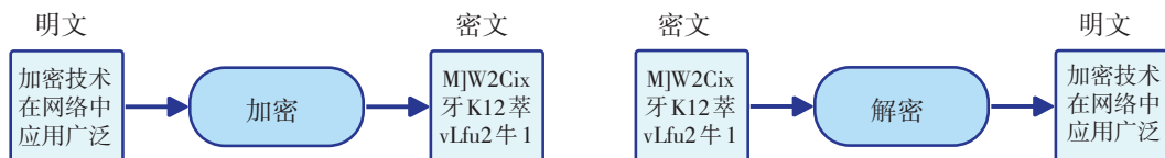
图3.1.10 加密与解密
