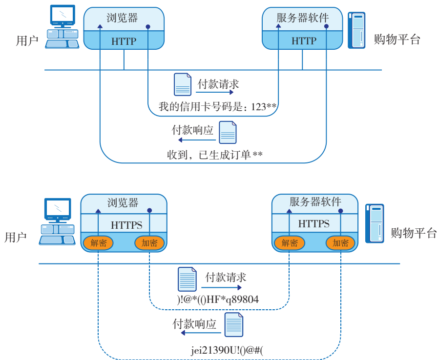
图 3.1.23 HTTP 与 HTTPS
