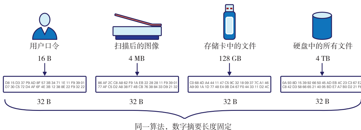
图 3.1.2 数字摘要
