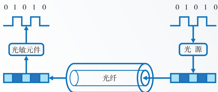
图 1.2.6 光纤通信原理示意图
