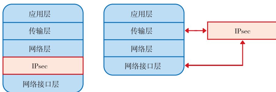
图 3.1.26 IPsec 的两种实现方式
